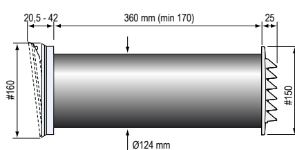
TL 80DE dBs - Bullerdämpande ventill
