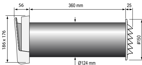
TL 80C dBs - Bullerdämpande ventill
