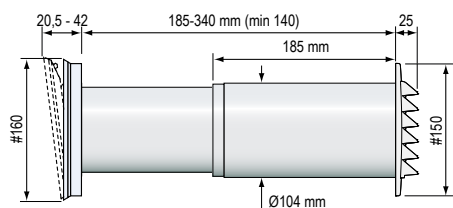
TL 100DE - Komplet ventill
