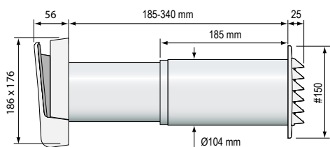
TL 100C - Komplet ventill
