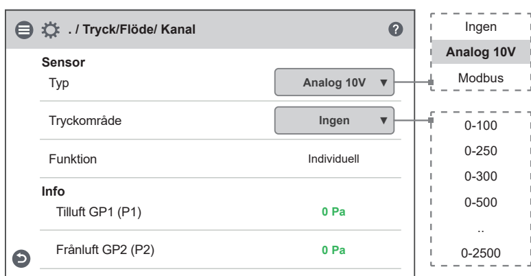
Service 1991 – Installation / Kringutrustning / Tryck/Flöde / Kanal – Analog 10V
