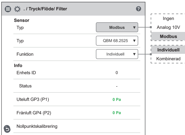
Service 1991 – Installation / Kringutrustning / Tryck/Flöde / Filter – Modbus
