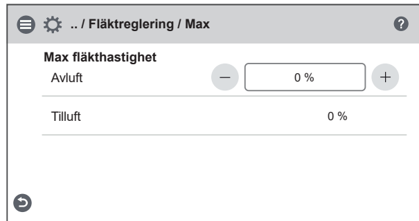
Wizard – 13.1 – Fläktinglering "%"/ Max fläkthastighet
