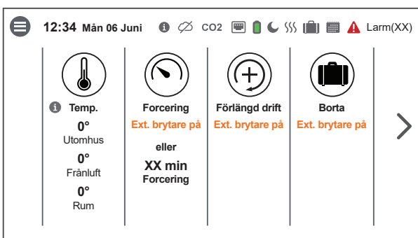
Hemskärm avancerad
