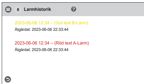
Larmhistorik
