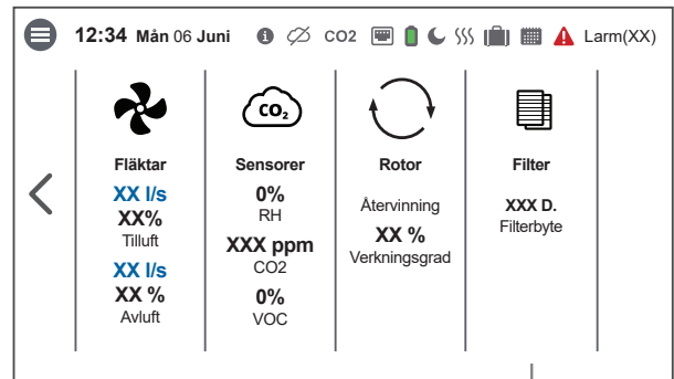
Hemskärm avancerad
