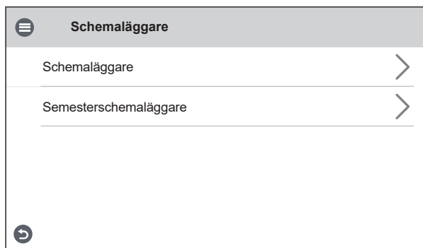
Schemaläggare meny
