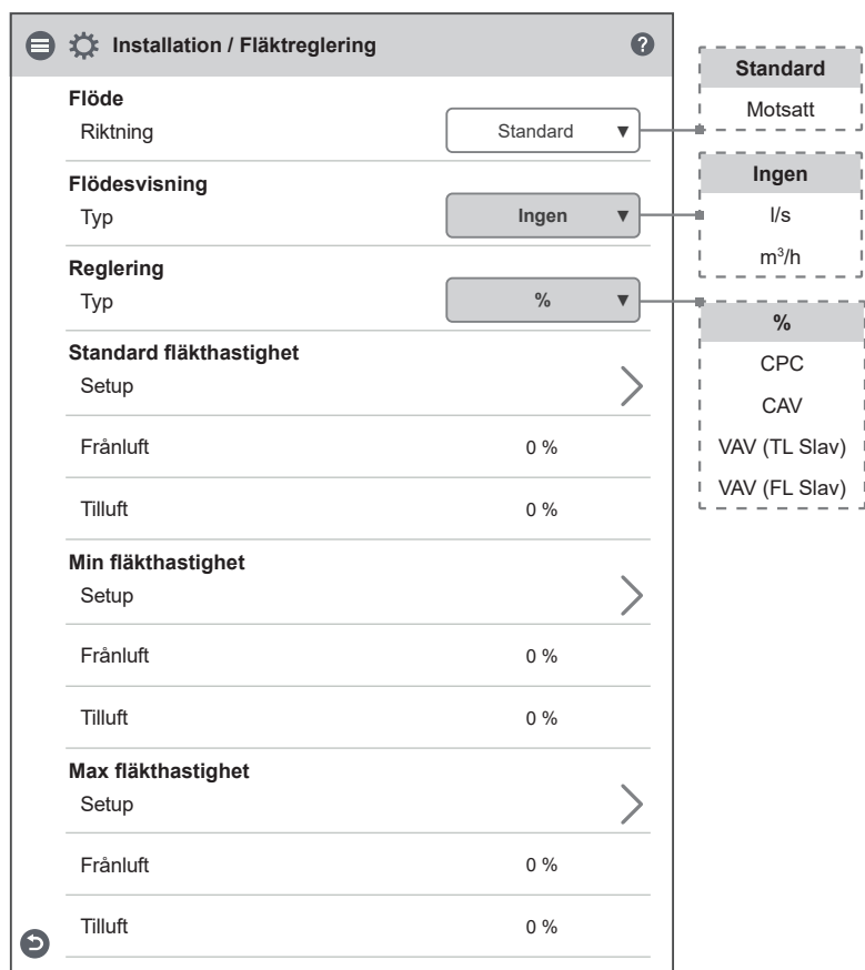
Service 1991 – Installation / Fläkttreglering "%"
