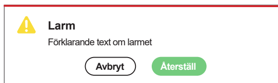
Återställ larm
