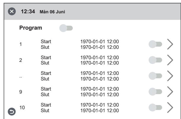
Semesterschemaläggare
