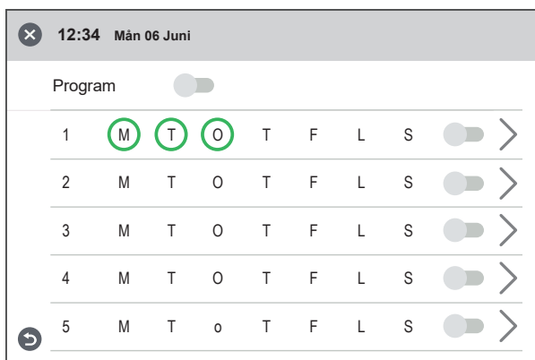
Veckoschemaläggare
