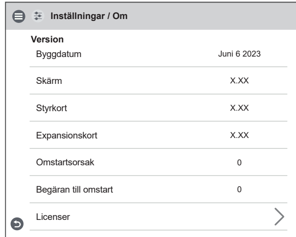
Inställningar – OM
