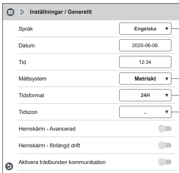
Inställningar generella
