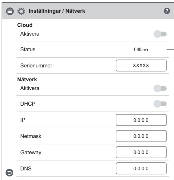
Inställningar – Nätverk
