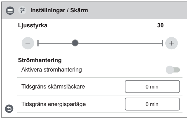
Inställningar – skärm
