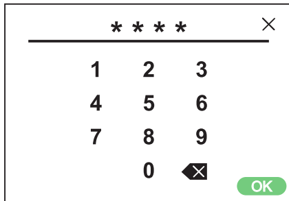
Serviceanvändare – kod 1199
