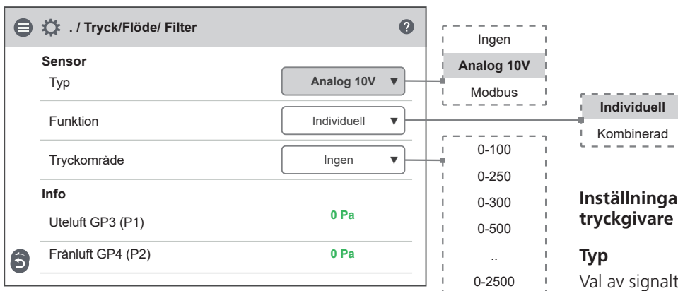
Service 1991 – Installation / Kringutrustning / Tryck/Flöde / Filter – Analog 10V
