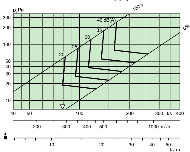
ALG 500-150 + TRG-B Ø250, Supply air
