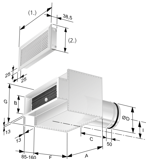
Figure 2. ALG/TRG. (1.) Nom. width + 30 mm (2.) Nom. height + 30 mm
