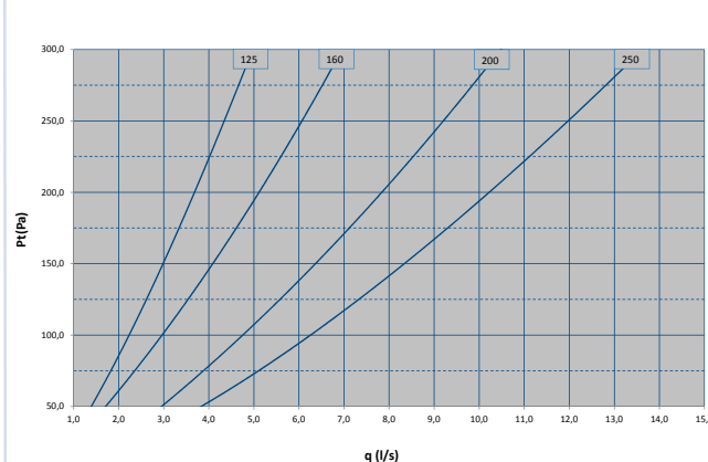
Diagram 6, läckage vid stängt spjäll Tellus-LÖV VAV
