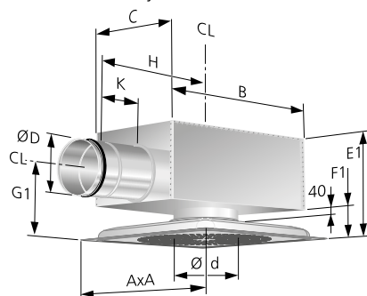
Figur 6. LOCKZONE Ceiling med ALS.
