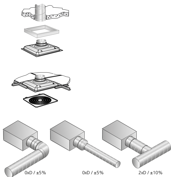
Figur 2. Monteringsalternativ.
