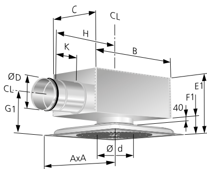
Figur 7. LOCKZONE C med ALS.
