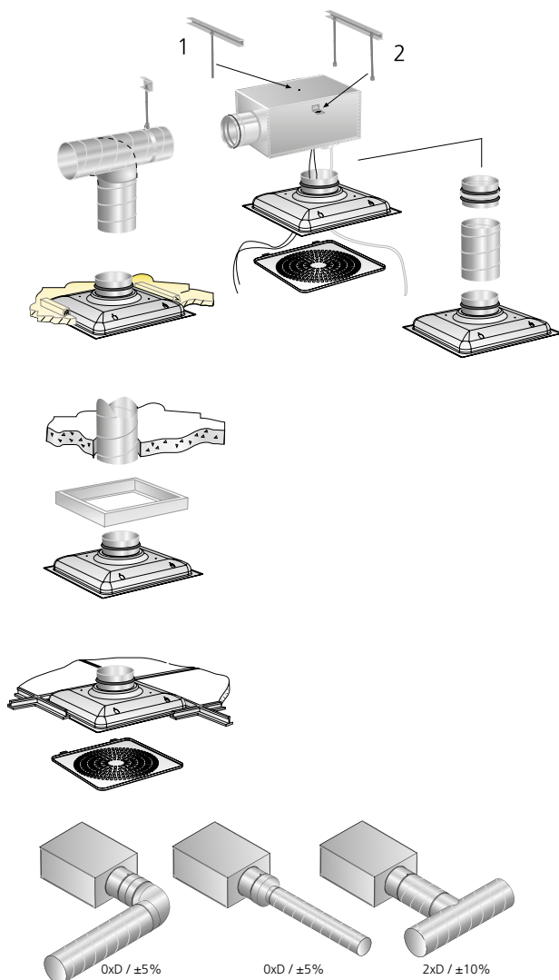
Figur 3. Monteringsalternativ.
