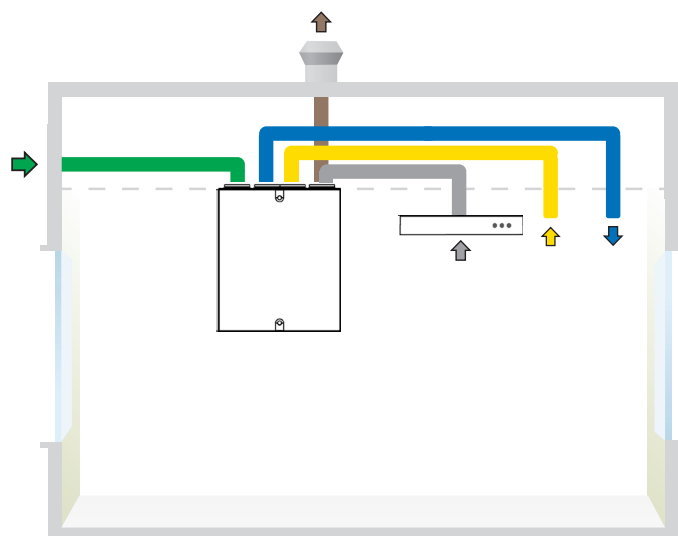
CASA R3 R, kanalanslutningar och spiskåpa anslutna till kökskanalanslutningen ovanpå ventilationsaggregatet.
