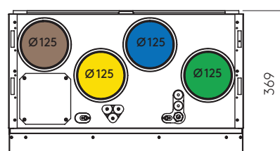
CASA R3 L Flat, vänsterutförande
