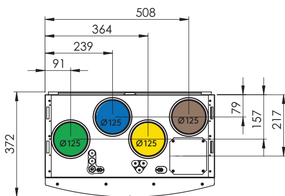
CASA R3 R, högerutförande
