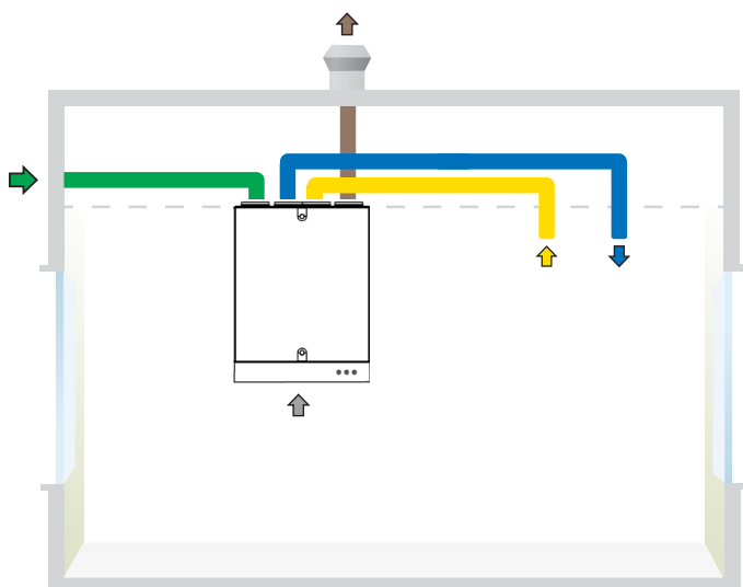
CASA R3 R, kanalanslutningar och spiskåpa anslutna till botten av ventilationsaggregatet.
