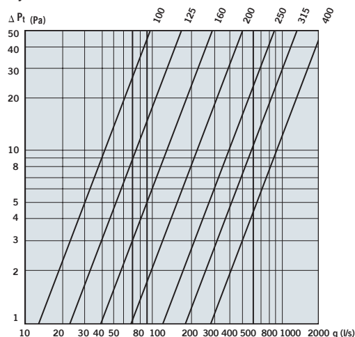
Tryckfall - Luftflöde
