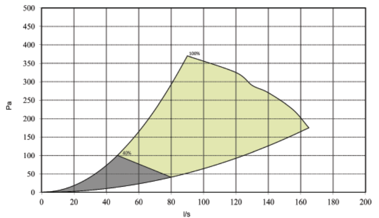
Luftflödesdiagram
