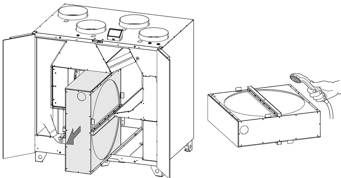
Fig. 6 Borttagning och rengöring av värmeväxlaren
