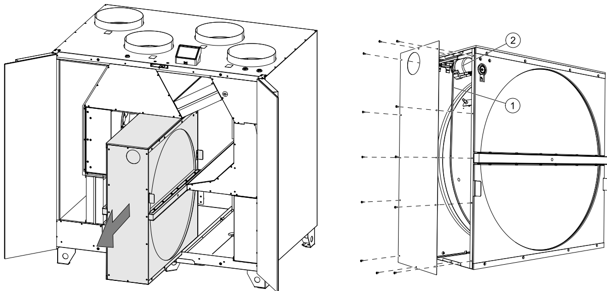
Bild 8 Zugang zum kaputten Rotor-Antriebsriemen
