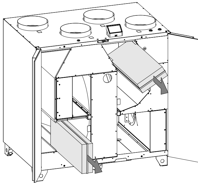
Kuva 5 Suodattimien vaihtaminen
