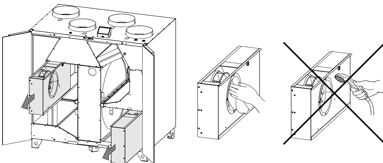
Fig. 7 Borttagning och rengöring av fläktar
