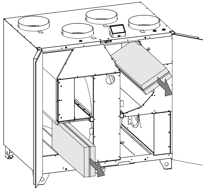
Fig. 5 Filterbyte
