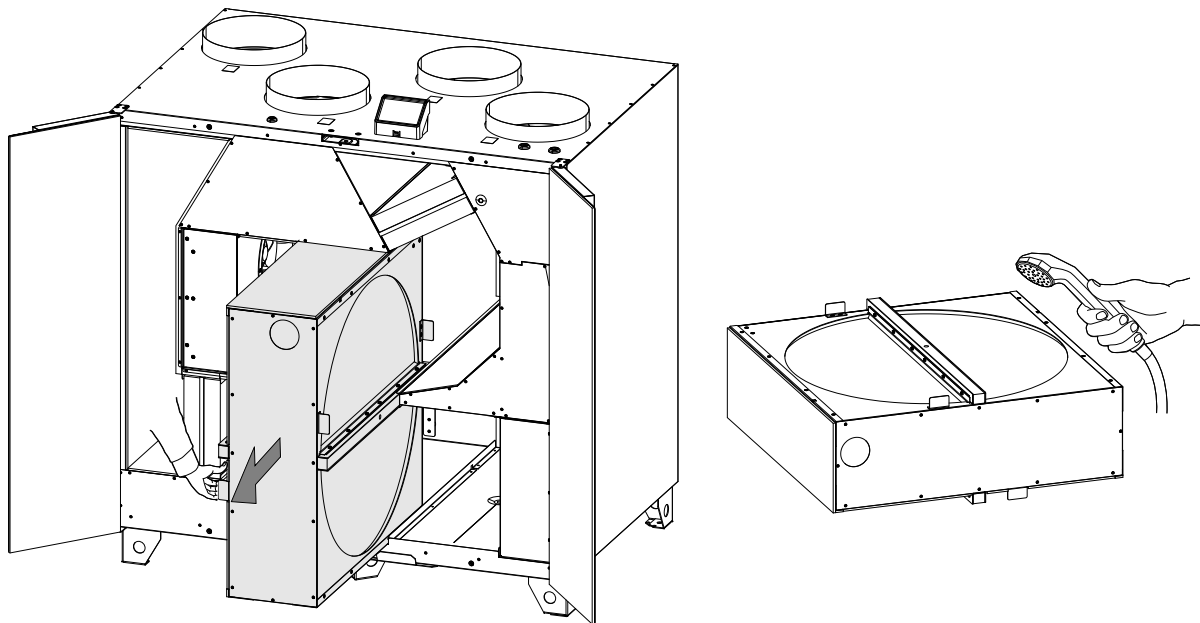
Bild 6 Entfernen und Reinigen des Wärmetauschers
