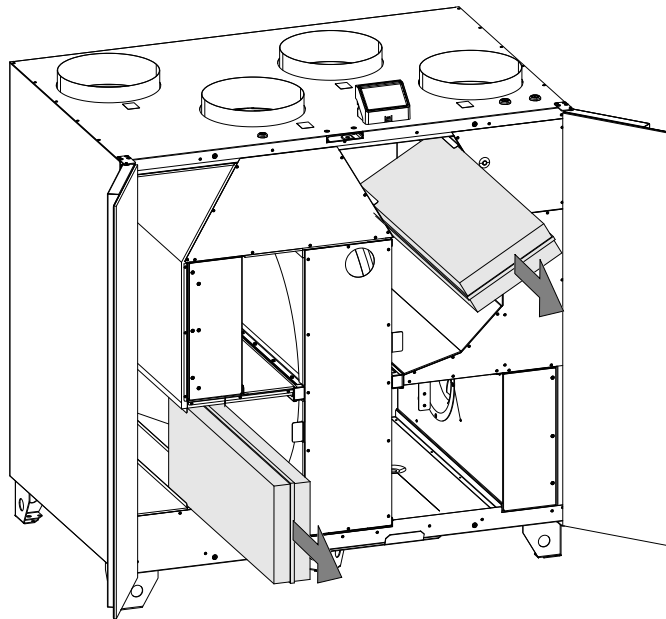
Bild 5 Auswechseln der Filter
