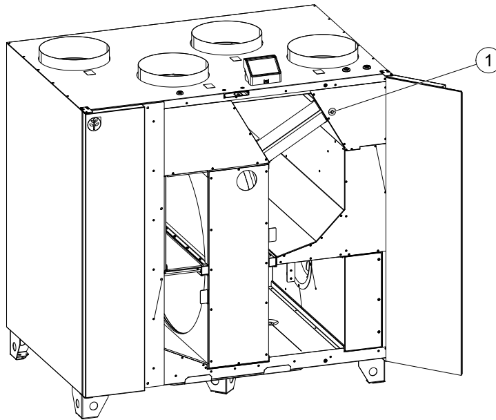
Kuva 9 Ylikuumenemisanturin palautuspainike
