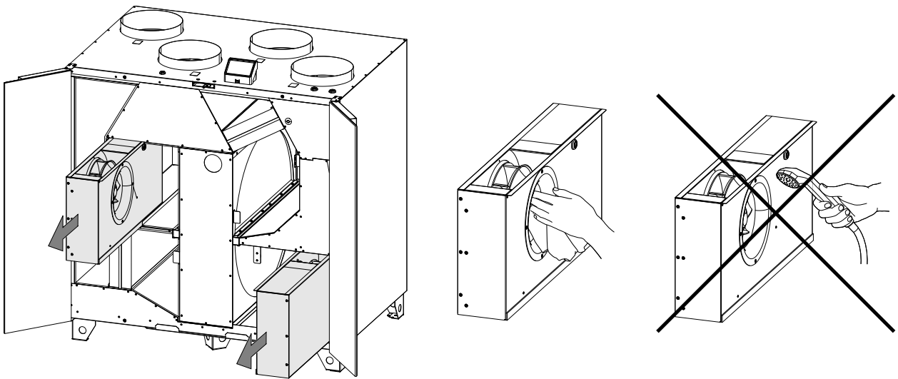
Bild 7 Entfernen und Reinigen der Lüfter
