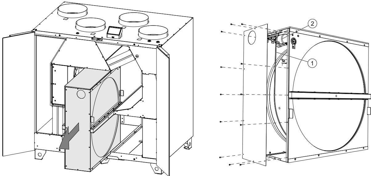
Kuva 8 Pääse käsiksi rikkoutuneeseen roottorin käyttöhihnaan
