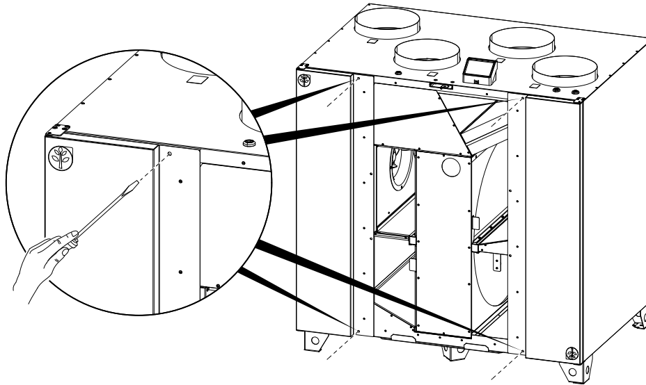
Kuva 4 Sivuvien avaus
