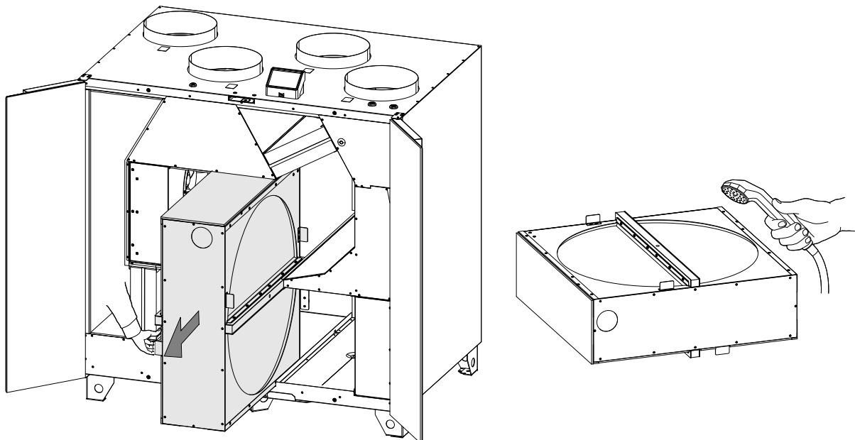
Kuva 6 Lämmönsiirtimen tarkastus ja puhdistus
