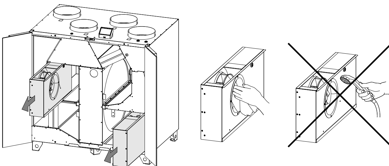
Kuva 7 Puhaltimien tarkastus ja puhdistus
