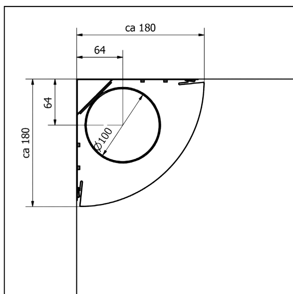
Ø100 under 125 panel med 125 fäste
