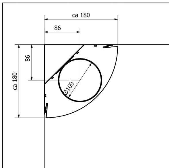
Ø100 under 125 panel med fäste 100
