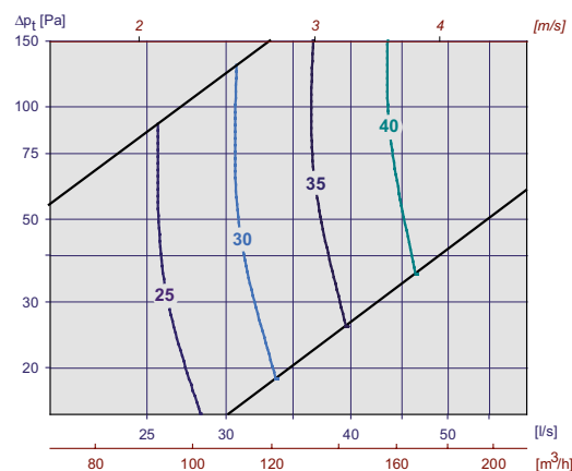
Diagram 4, TLG-LÖV m/Luna 125-125
