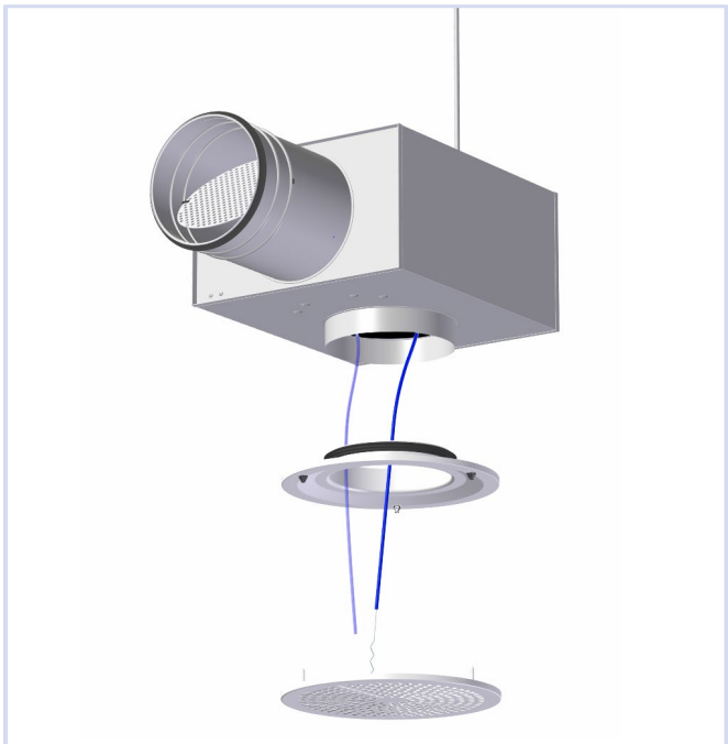
Bild 5, montage
