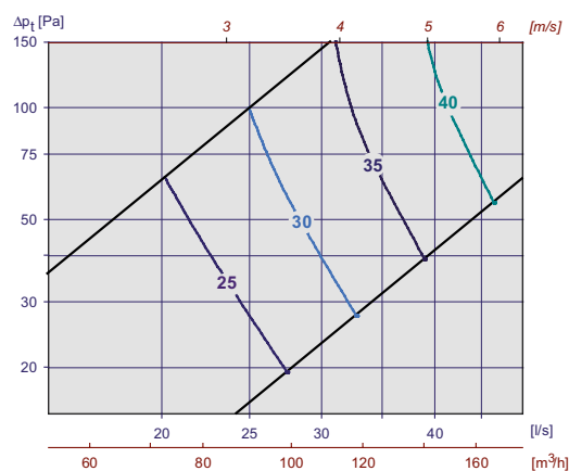
Diagram 2, TLG-LÖV m/Luna 100-125
