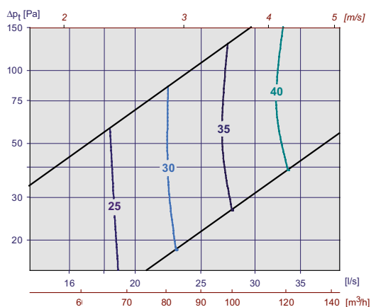
Diagram 1, TLG-LÖV m/Luna 100-100
