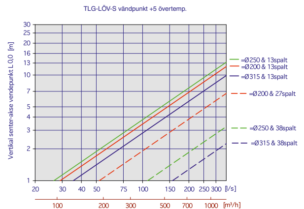
Diagram 20, +5° övertemperatur.
