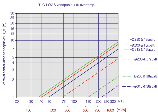
Diagram 21, +10° övertemperatur.
