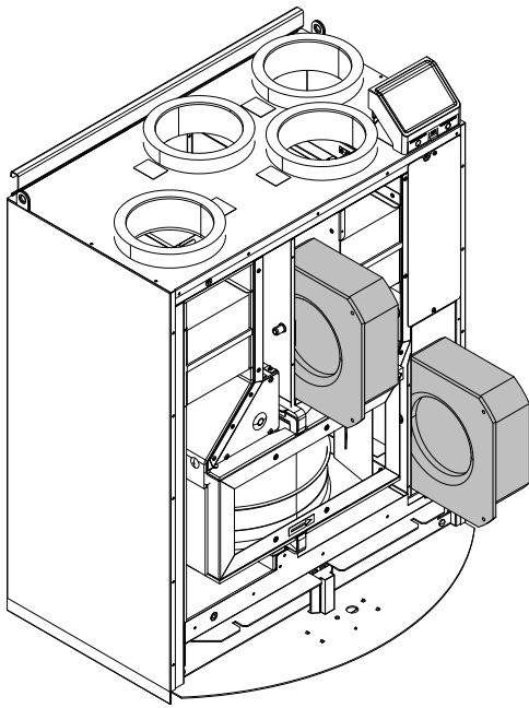
Bild 9 Abluft- und Zuluftventilatoren
