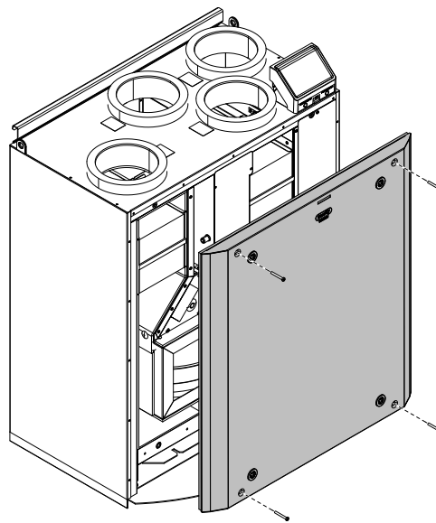
Bild 6 Innere Abdeckung entfernen / befestigen
