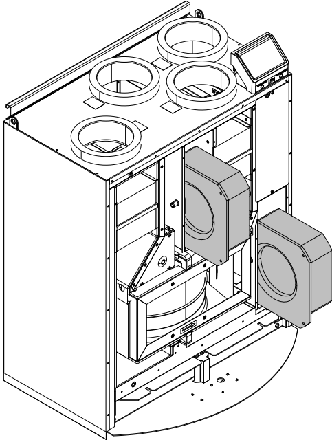
Fig. 9 Från- och tilluftsfläktar
