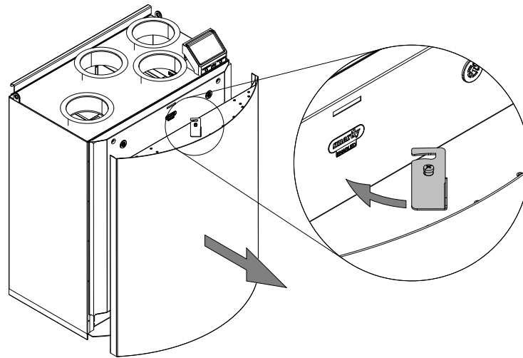
Bild 5 Äußere Frontabdeckung entfernen / befestigen
