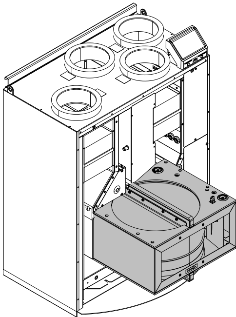
Kuva 8 Lämmönvaihdin
