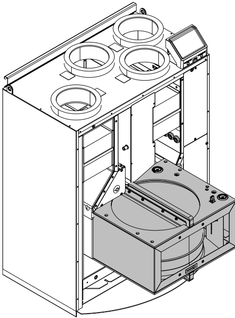
Bild 8 Wärmetauscher
