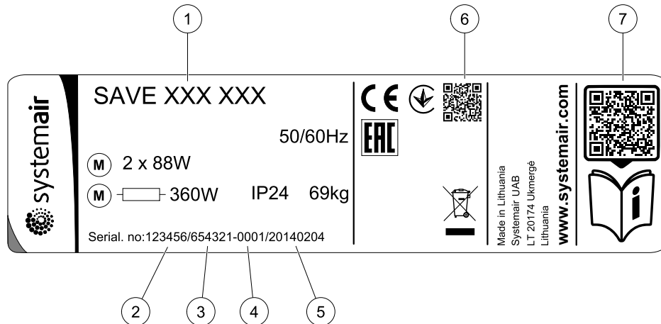
Kuva 1 Laitekilpi
