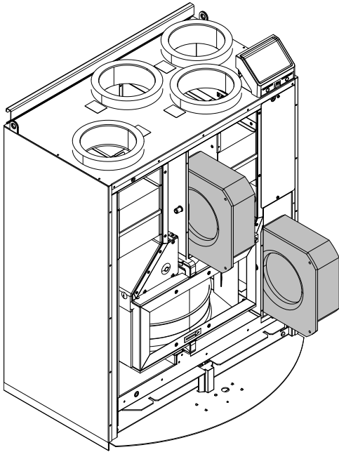
Kuva 9 Poisto- ja tuloilmapuhaltimet
