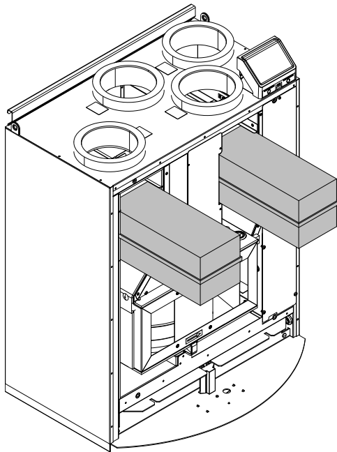
Fig. 7 Värmeväxlarfilter
