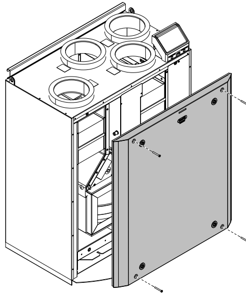
Kuva 6 Etulevyn irrotus/asennus
