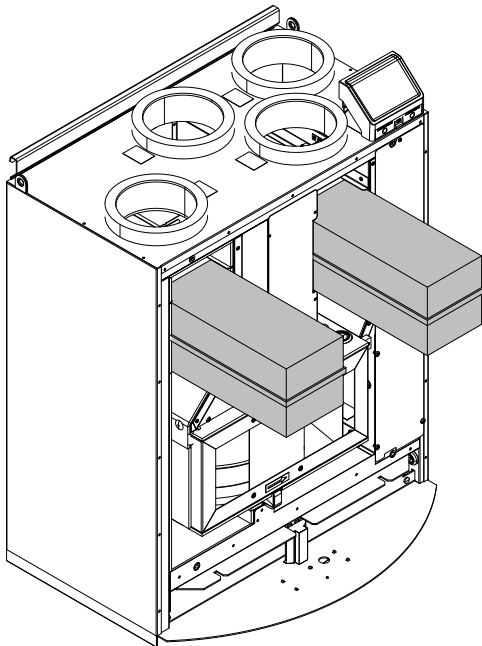
Bild 7 Wärmetauscherfilter
