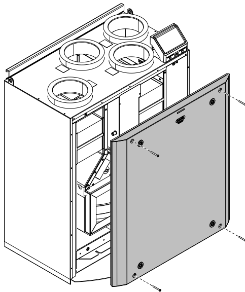
Fig. 6 Demontering/montering av invändig front
