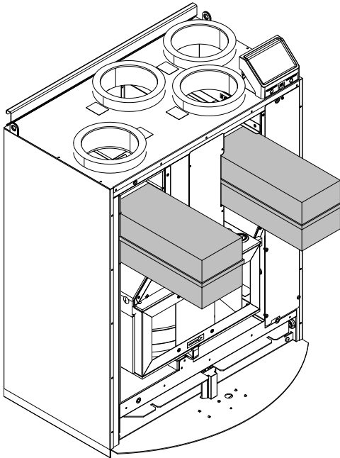
Kuva 7 Lämmönsiirtimen suodattimet
