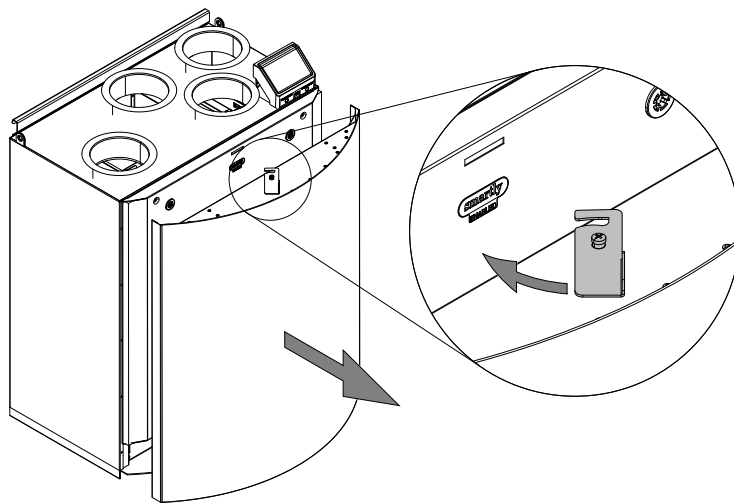
Fig. 5 Demontering/montering av utvändig front
