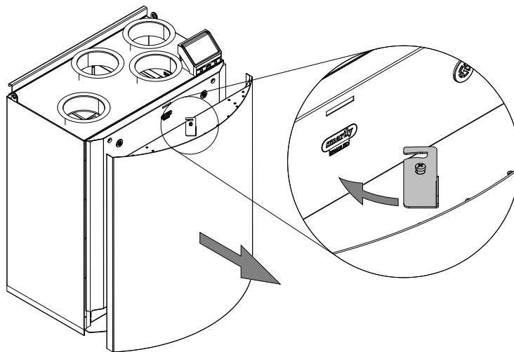
Kuva 5 Etupaneelin irrotus/asennus
