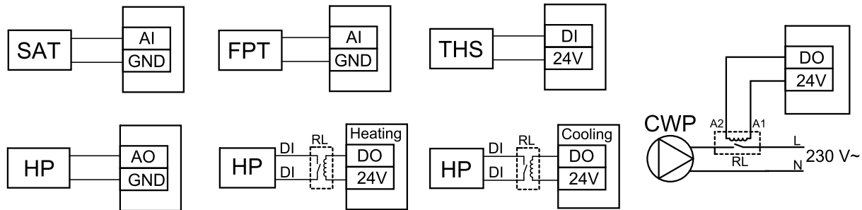
Kuva 19 Yhdistelmäpatterin liitännät
