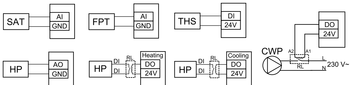
Bild 19 Anbindung DX-Heiz-/Kühlregister
