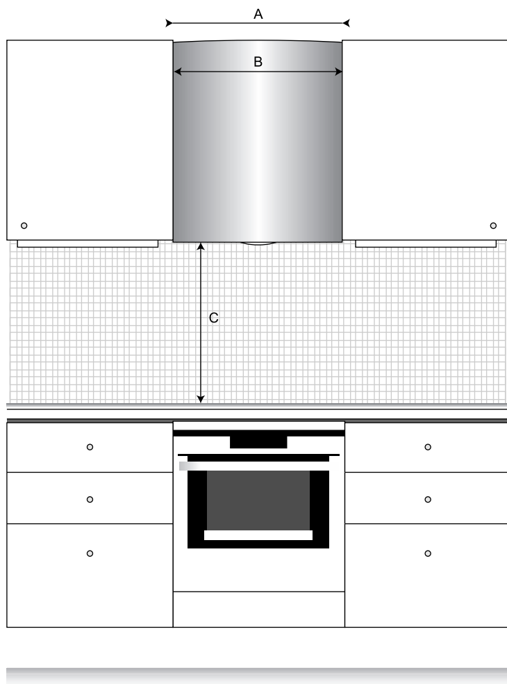
Kuva 3 SAVE VTR 150/K keittiöympäristössä
