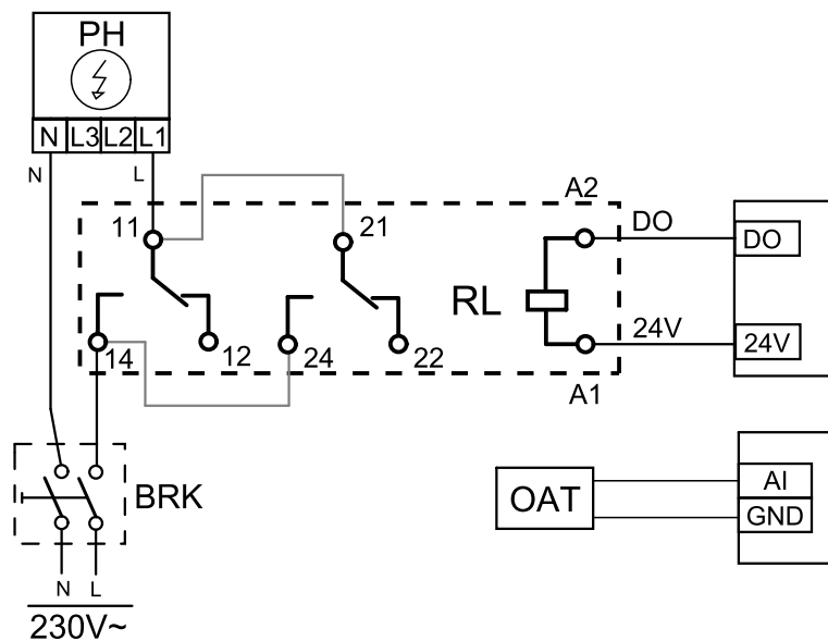
Fig. 16 Fövärmanslutningar
