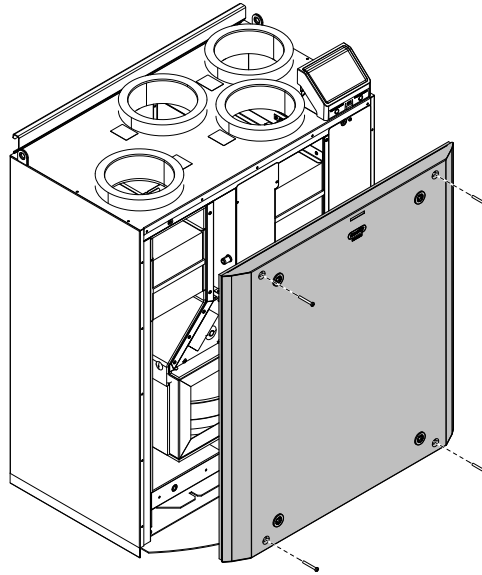
Kuva 5 Etulevyn irrotus/asennus
