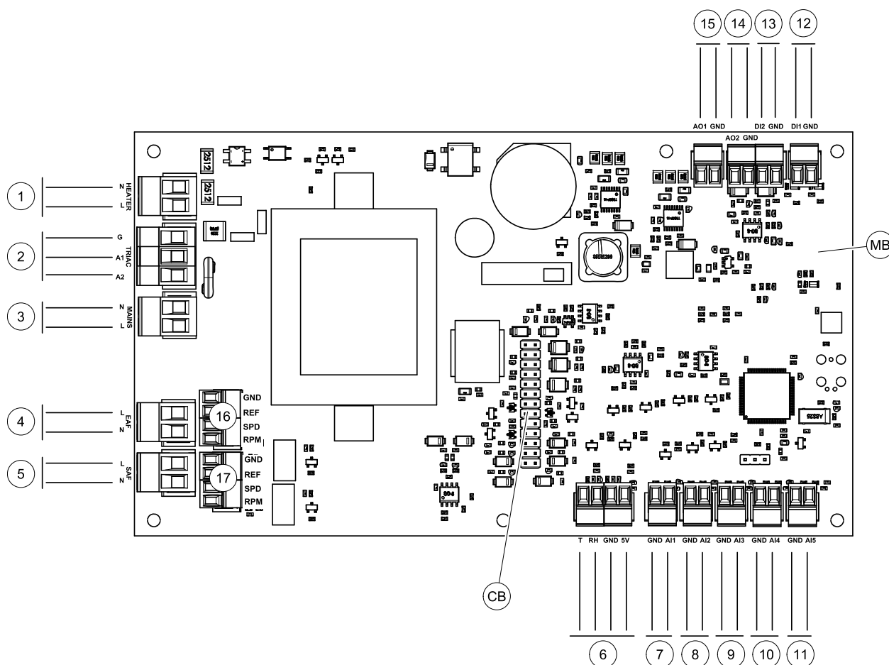
Fig. 10 Huvudkretskortet anslutningar
