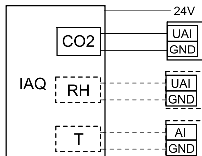
Kuva 15 IAQ liitännät
