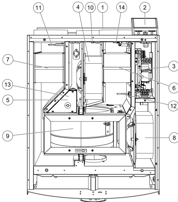
Bild 12 Interne Komponenten
