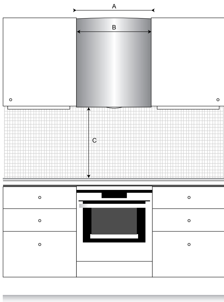
Bild 3 SAVE VTR 150/K in einer Küche
