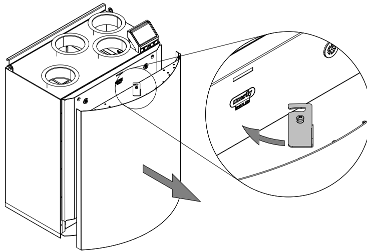
Bild 4 Äußere Frontabdeckung entfernen / befestigen
