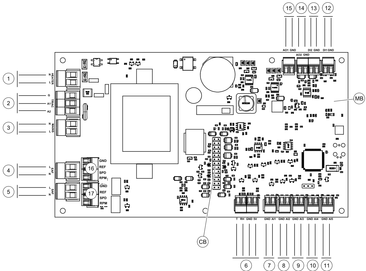
Bild 10 Anschlüsse der Hauptplatine
