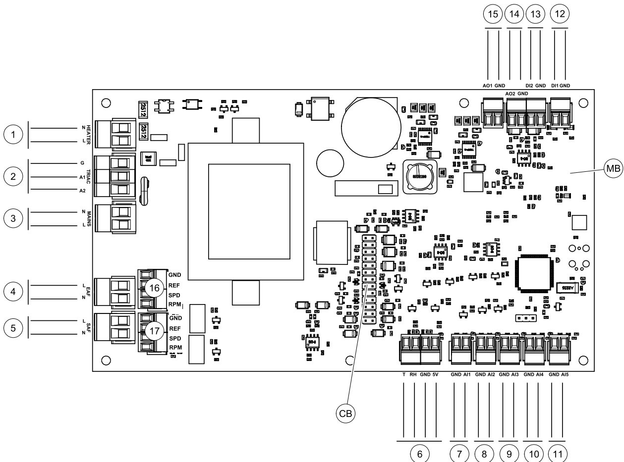
Kuva 10 Pääpiirilevyn liitännät
