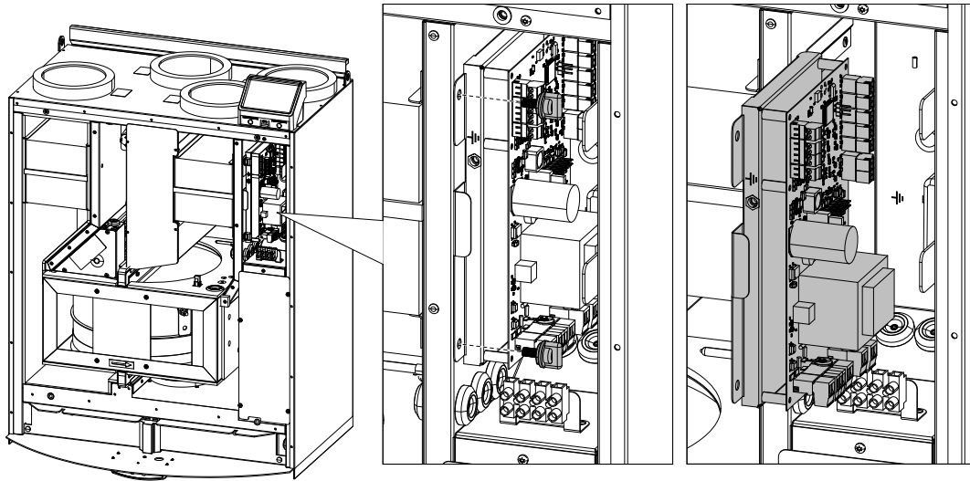
Kuva 9 Pääpiirilevyn sijainti
