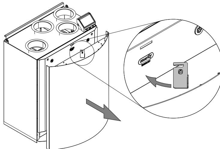
Kuva 4 Etupaneelin irrotus/asennus
