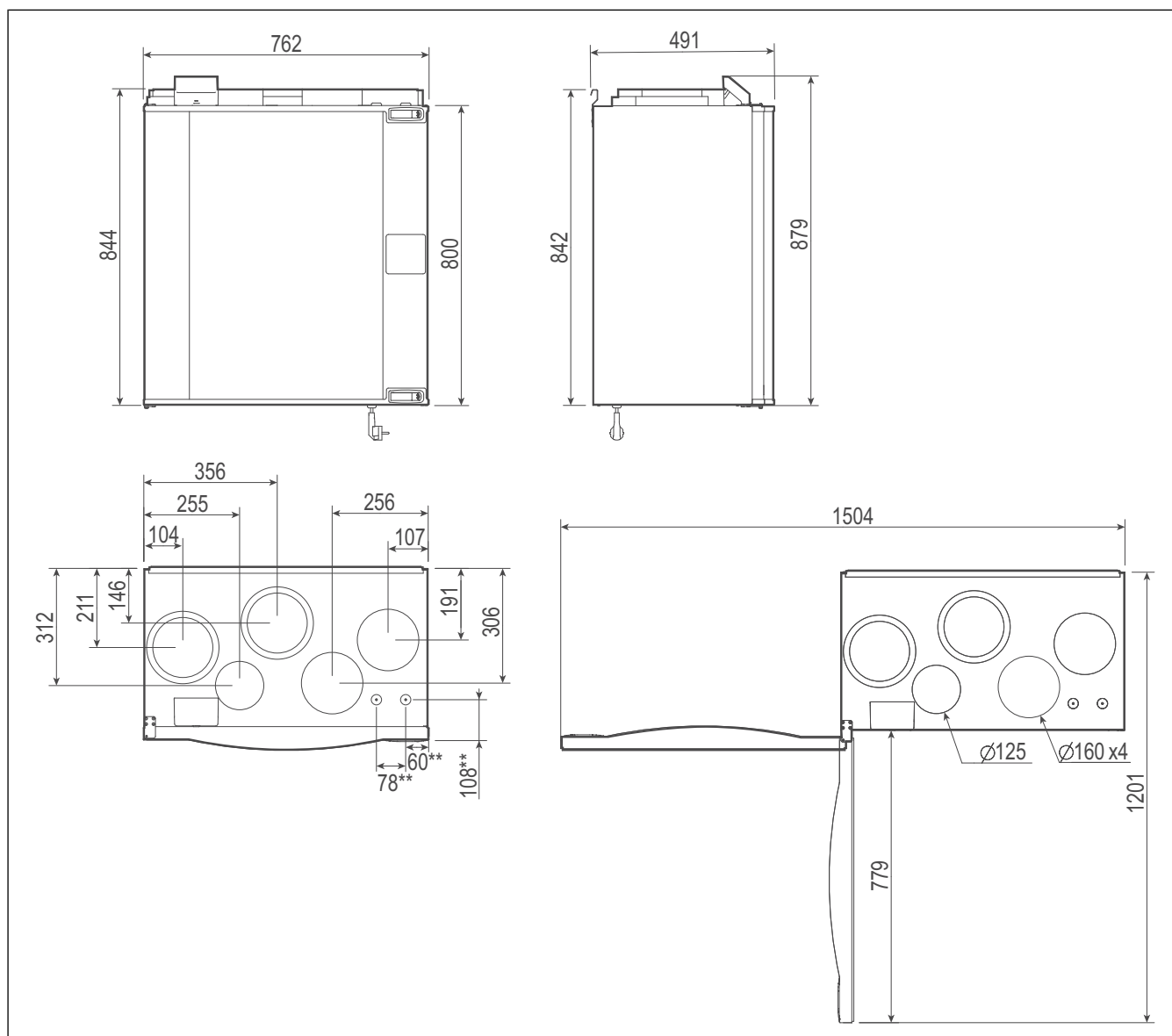
Fig. 2 Högermodell (tilluftsanslutning på höger sida)
