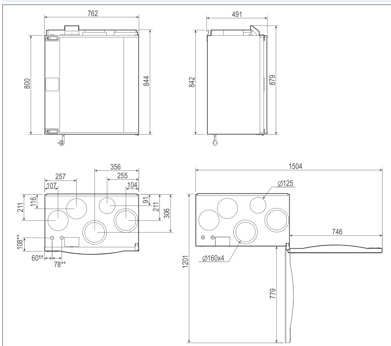
Fig. 1 Vänstermodell (tilluftsanslutning på vänster sida)
