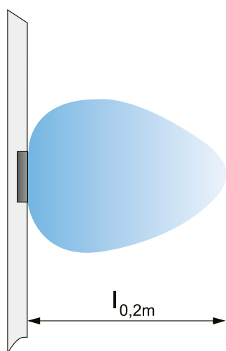
Figur 7. Isovel. Spridningsbild standard, kort kastlängd.
