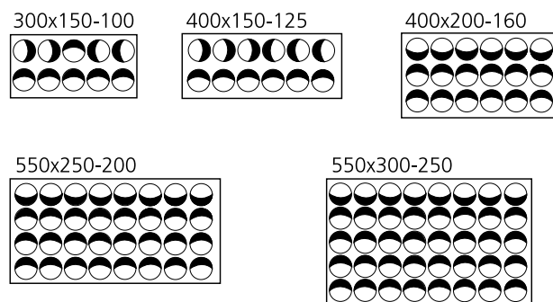
Figur 6. Standard dysmönster, lång kastlängd.
