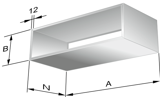
Figur 3. Täckplåt ALVT 1.
