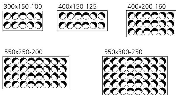
Figur 5. Standard dysmönster, kort kastlängd.
