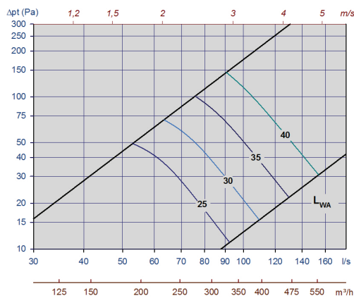
Diagram 11, Tellus-Opus-200-mitt.spalthöjd
