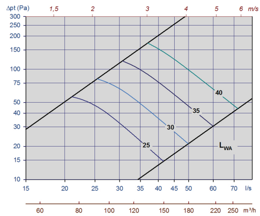
Diagram 6, Tellus-Opus-125-max.spalthöjd
