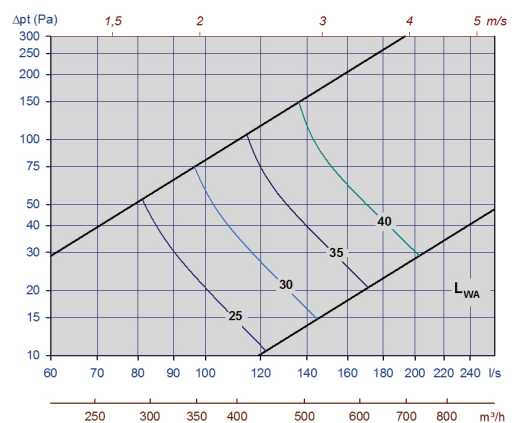
Diagram 14, Tellus-Opus-250-mid.spalthöjd
