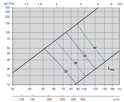
Diagram 10, Tellus-Opus-200-min.spalthöjd
