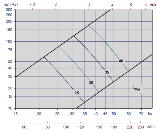
Diagram 4, Tellus-Opus-125-min.spalthöjd
