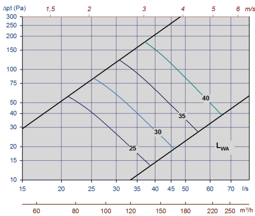
Diagram 5, Tellus-Opus-125-mitt spalthöjd
