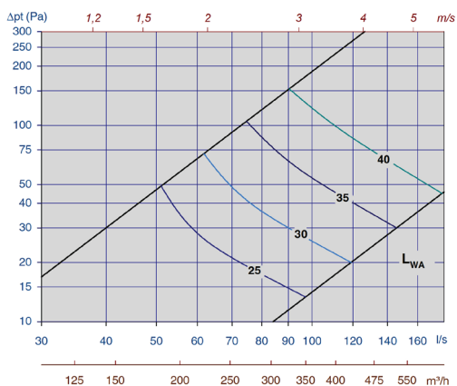
Diagram 19, Tellus-D-Opus-200-min. spalthöjd
