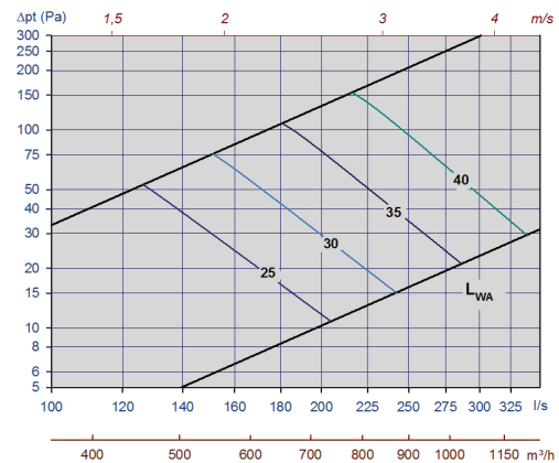
Diagram 18, Tellus-Opus-315-max. spalthöjd
