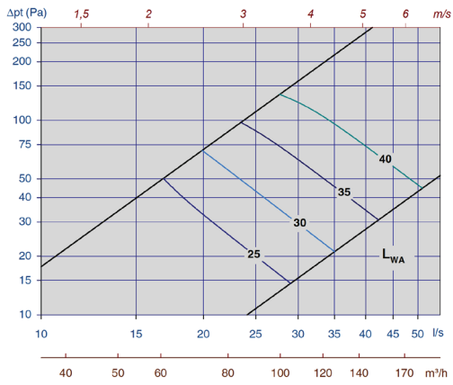
Diagram 3, Tellus-Opus-100-max.spalthöjd
