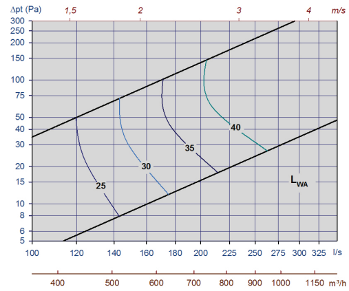
Diagram 16, Tellus-Opus-315-min. spalthöjd
