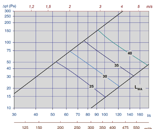
Diagram 20, Tellus-D-Opus-200-mitt spalthöjd
