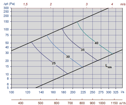
Diagram 17, Tellus-Opus-315-mitt spalthöjd
