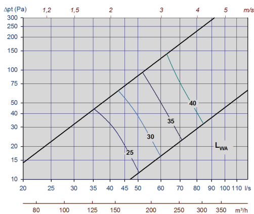
Diagram 7, Tellus-Opus-160-min.spalthöjd
