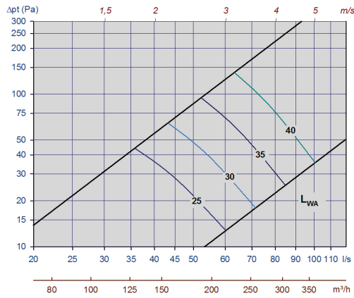
Diagram 9, Tellus-Opus-160-max.spalthöjd
