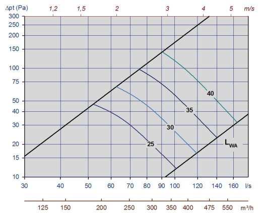
Diagram 12, Tellus-Opus-200-max.spalthöjd
