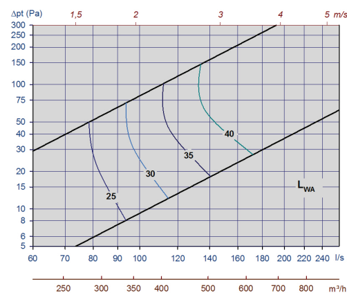
Diagram 13, Tellus-Opus-250-min.spalthöjd
