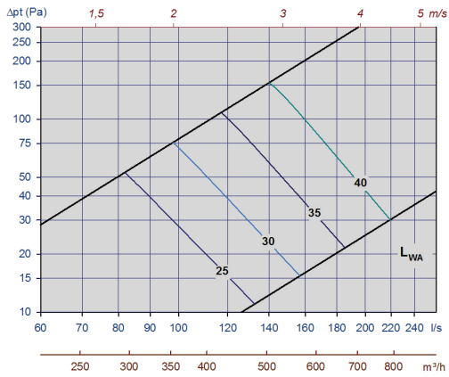
Diagram 15, Tellus-Opus-250-max. spalthöjd
