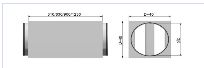
Bild 3, LKR med ljuddämpande baffel > \varnothing 315
