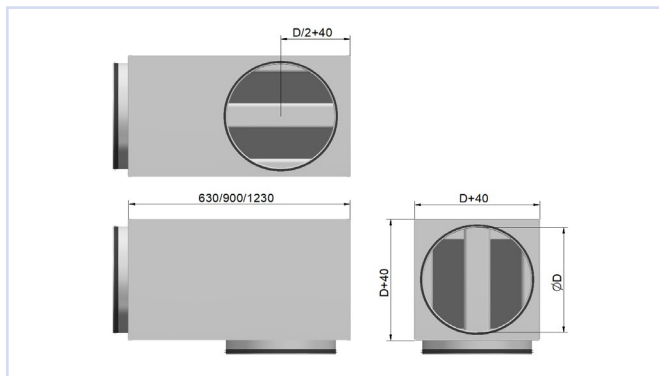
Bild 4, LKR-V med ljuddämpande baffel > \varnothing 315
